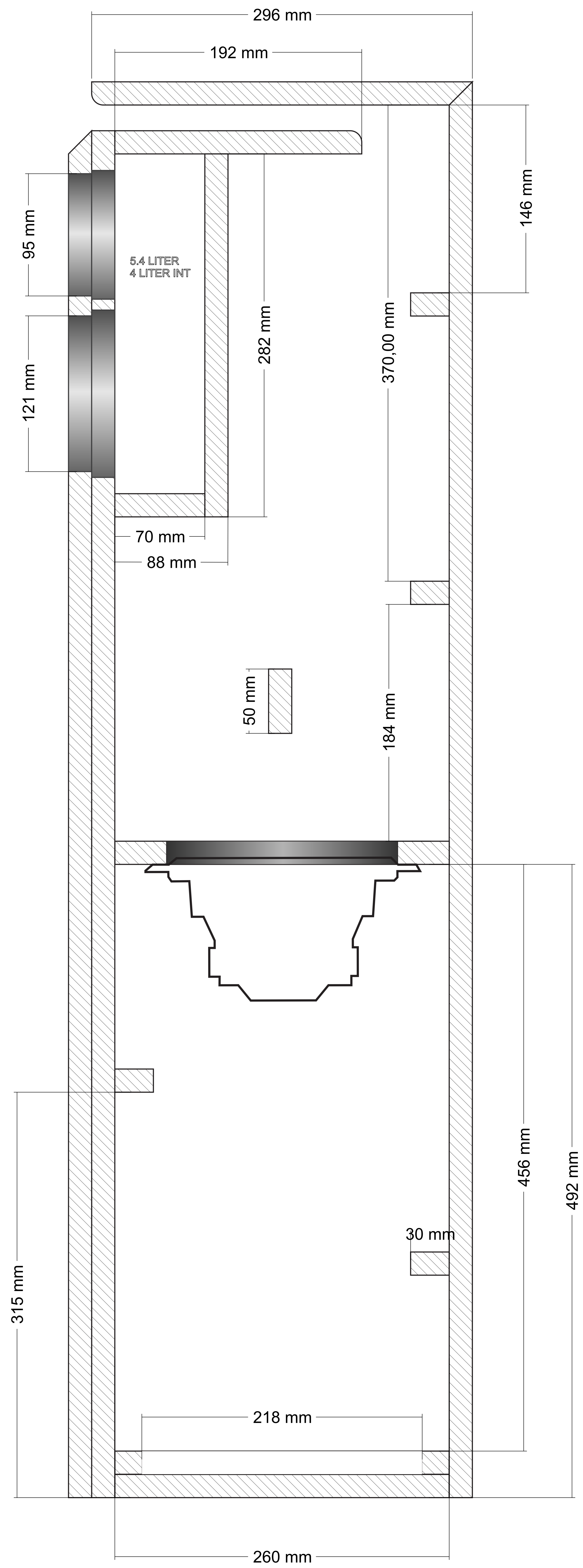
Zij aanzicht
